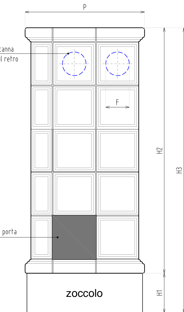
VISTA LATERALE
