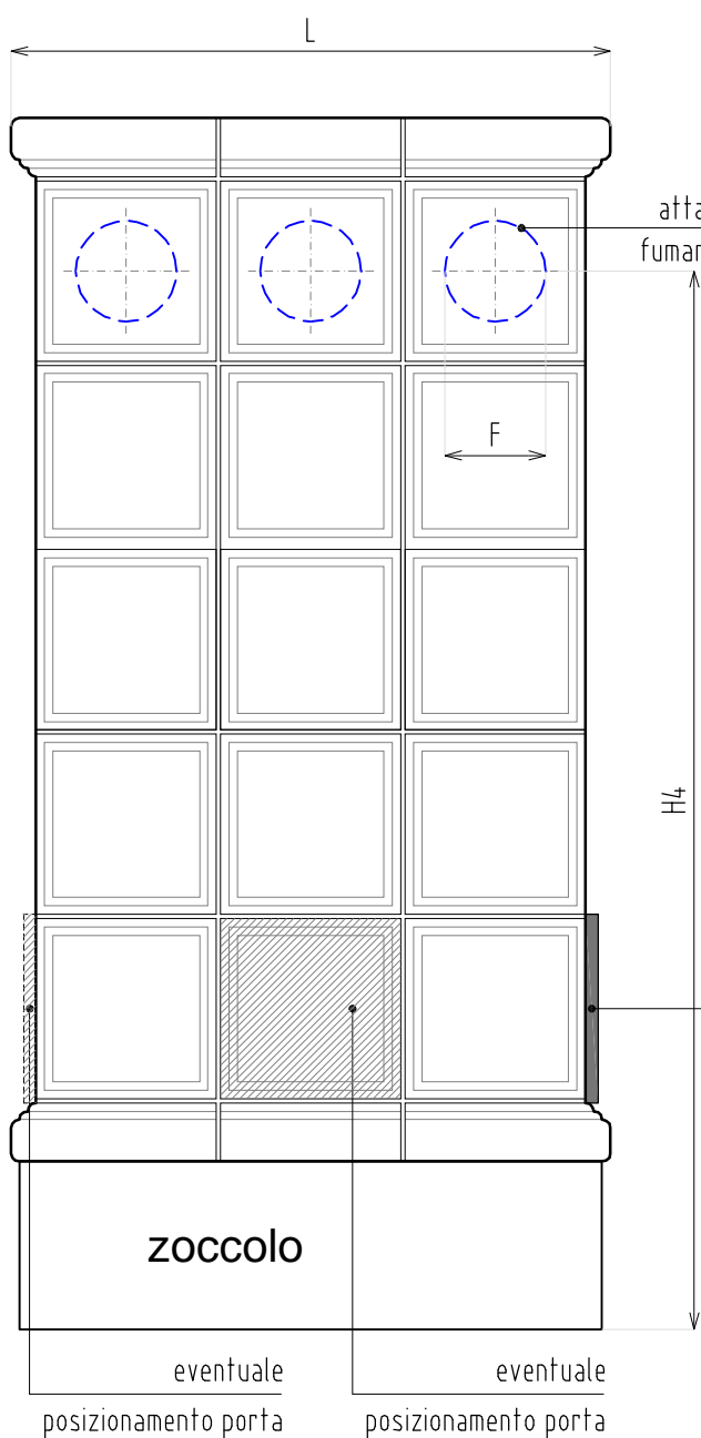
VISTA FRONTALE
