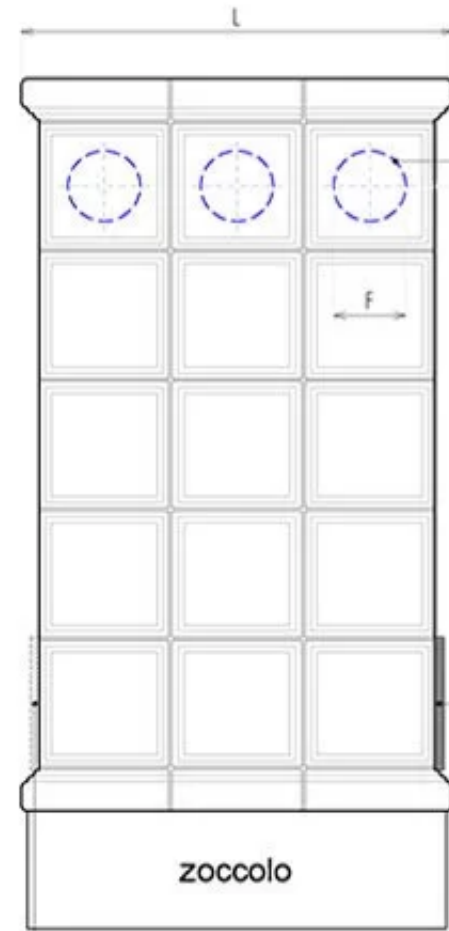
VISTA FRONTALE
