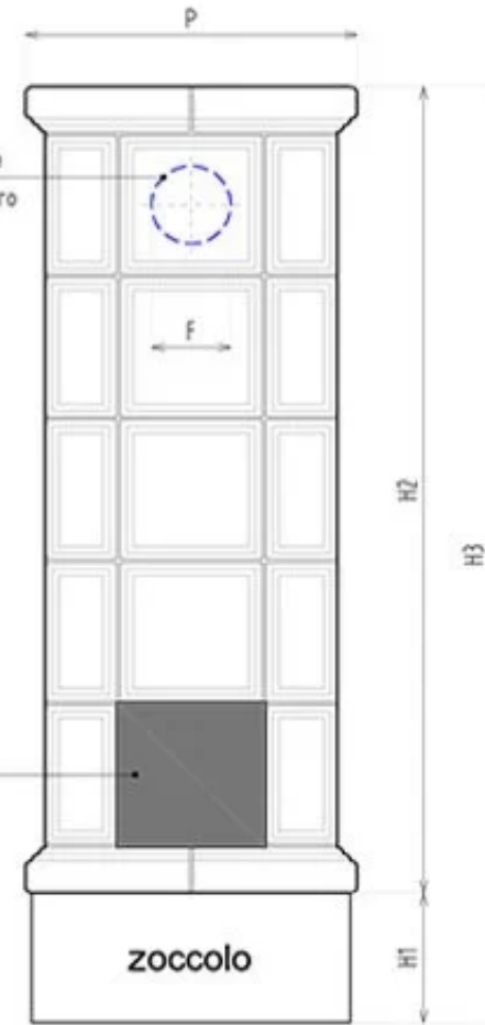
VISTA LATERALE
