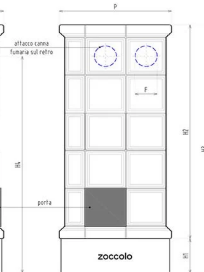
VISTA LATERALE
