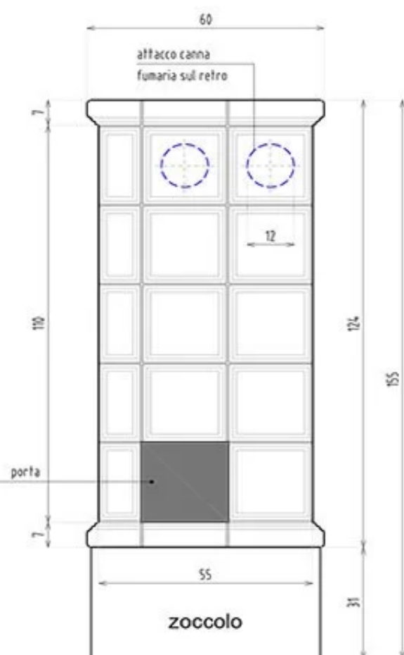
VISTA LATERALE
