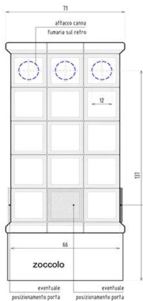
VISTA FRONTALE
